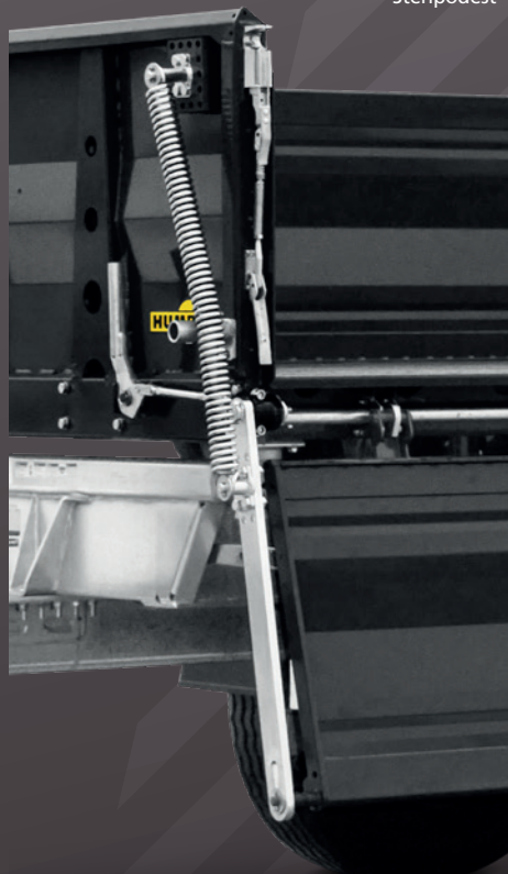
Seitenbordwand abklappbar mit Federentlastung
